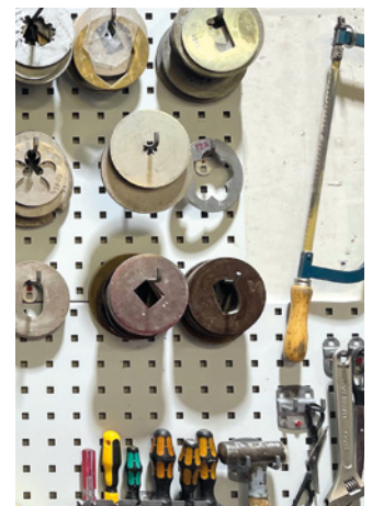
Ziehmatrizen
